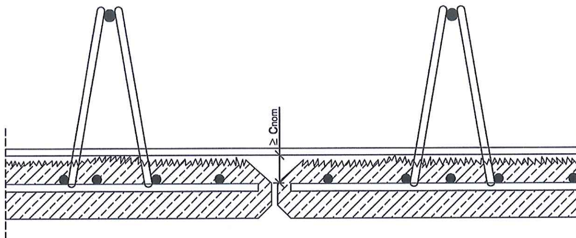
Bild 5: Abfasung an Elementrändern
