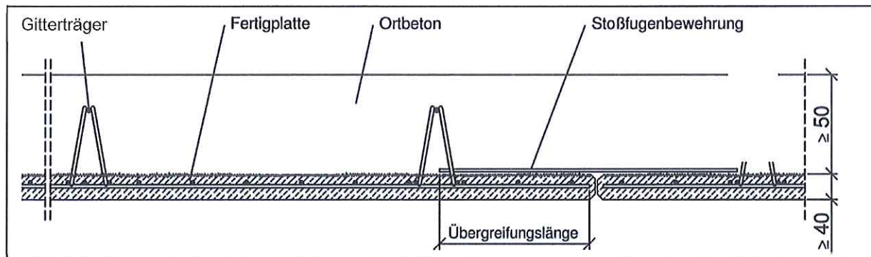
Bild 2: Beispiel Elemente mit Betonstahlmatten
